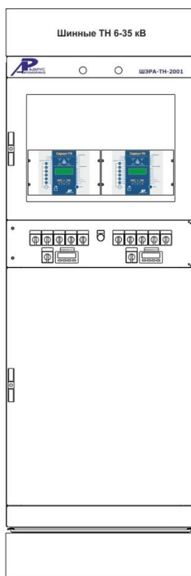
Шкаф шинных ТН 6-35 кВ ШЭРА-ТН-2001 БПВА.656457.455, БПВА.650645.001 ТУ
